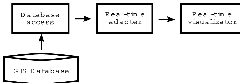
Figura 6: Arquitectura global para datos vectoriales
